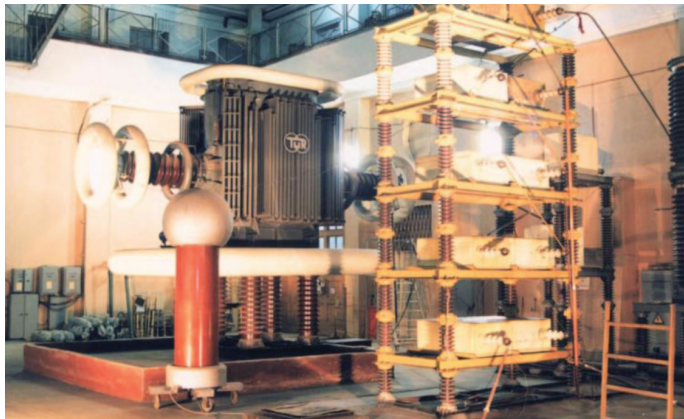
Рис. 6. Комбинированная испытательная установка переменного напряжения 500 кВ, 6 А и постоянного напряжения 500 кВ, 0,3 А
