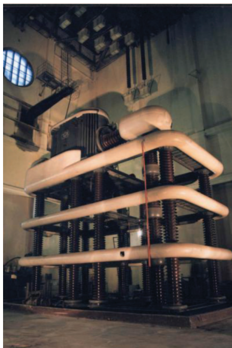
Рис. 4. Испытательный трансформатор 750 кВ, 2 А
